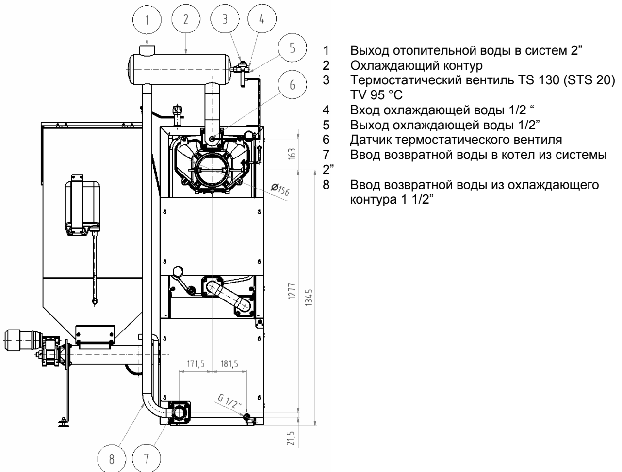
Рис. 3 Охлаждающий контур
