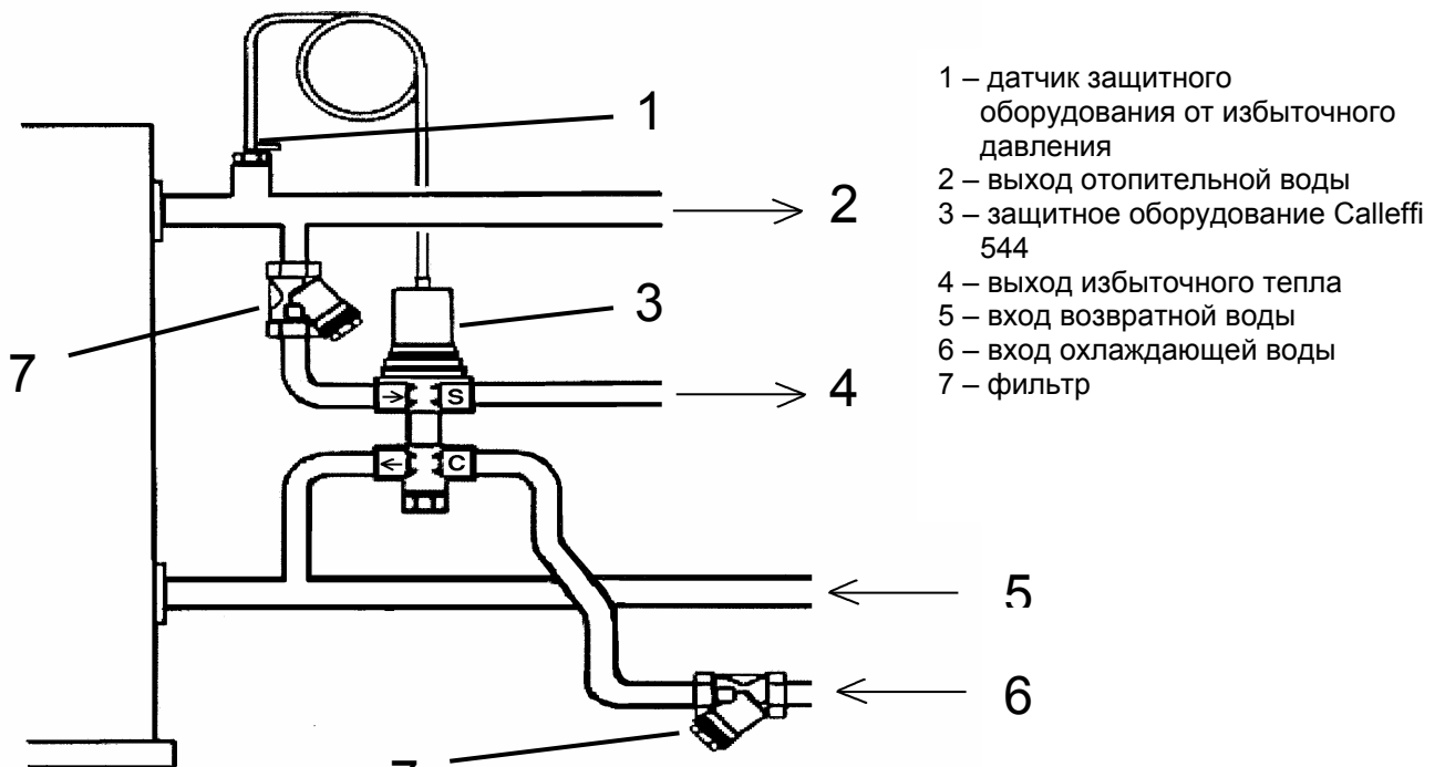
Рис. 5б) Гидравлическая схема
