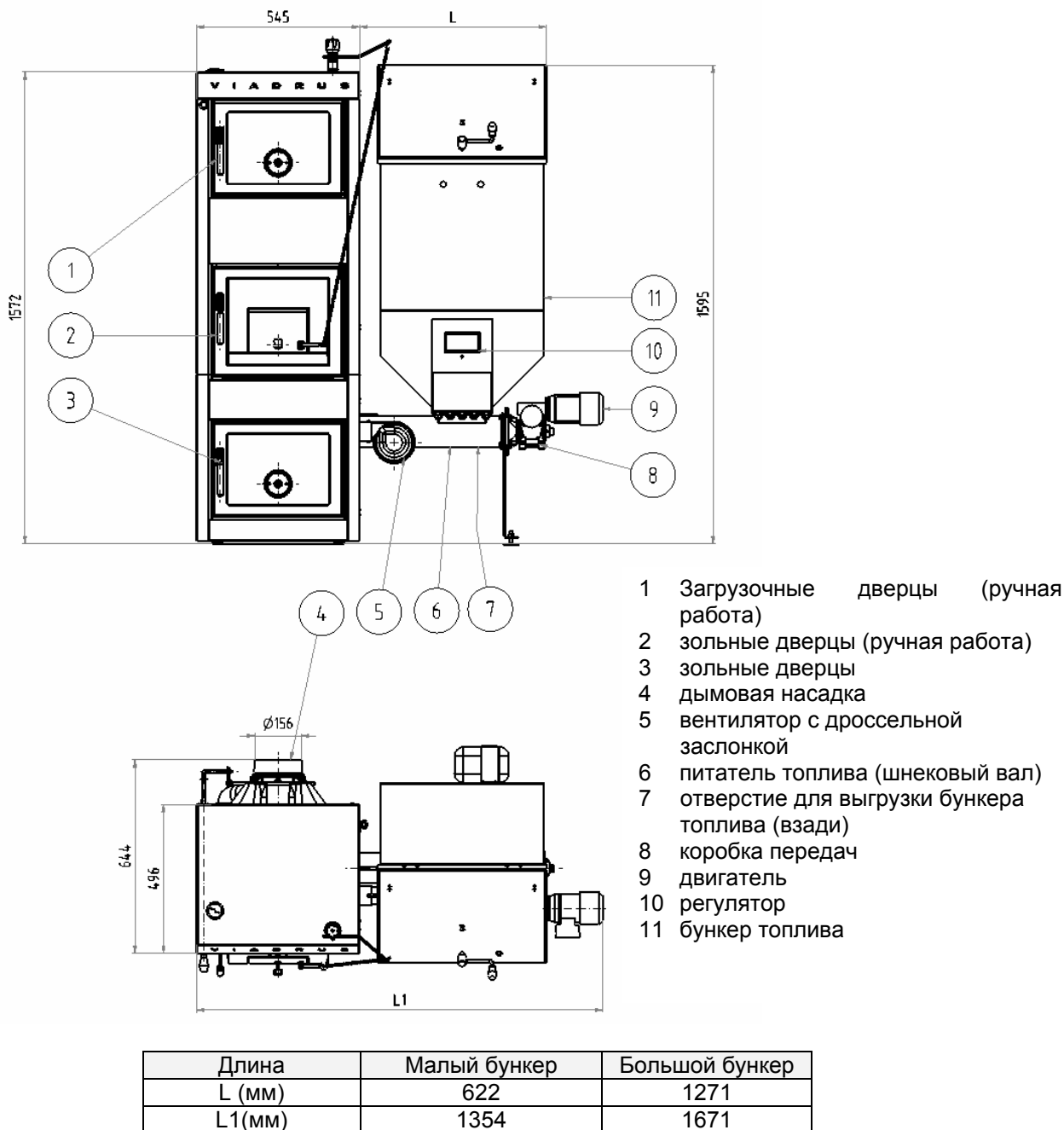
Рис. 1 Схема котла VIADRUS HERCULES DUO (правая версия)
