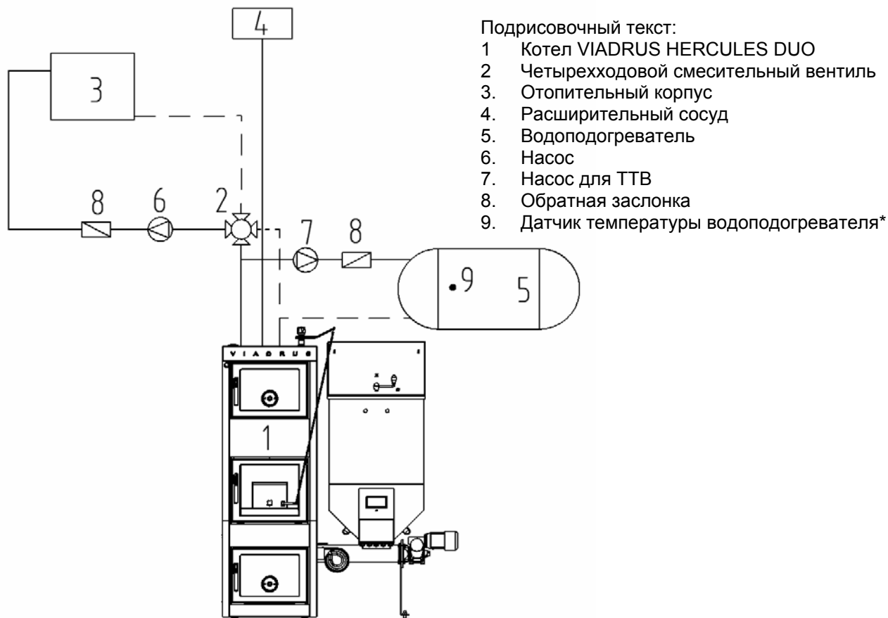
Рис. 10 Блок-схема установки ЦО в системе с четырехходовым вентилем
