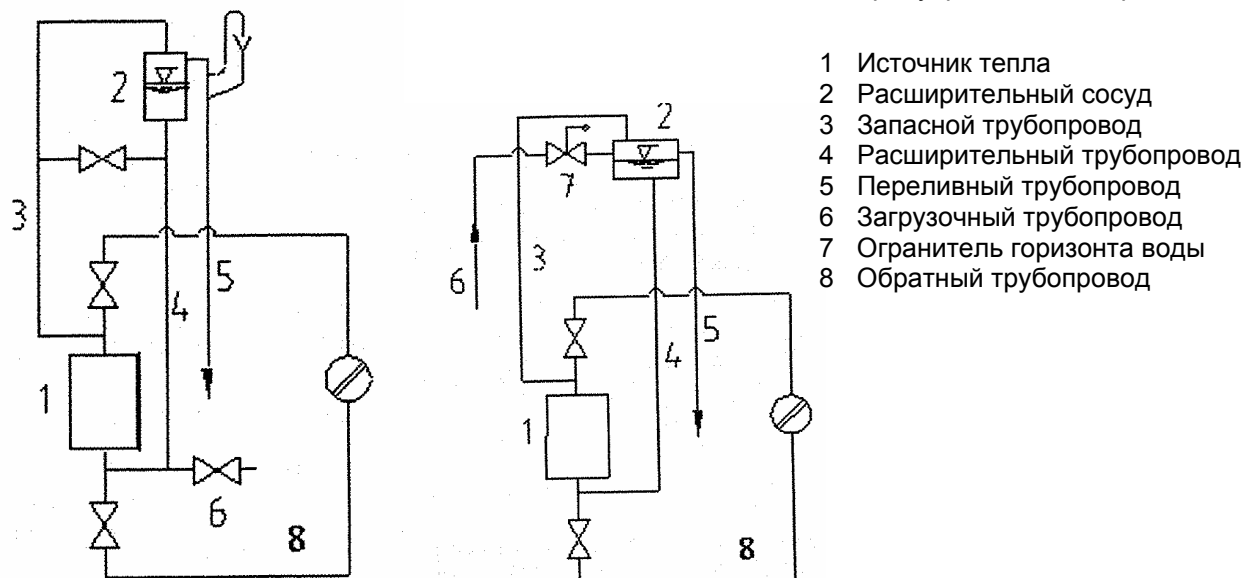
Рис. 6 Образцы подключения открытых расширительных сосудов
